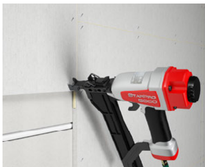
Bevestiging van de bijkomende laag fermacell® gipsvezelplaat of Powerpanel H 2 O incl. voegverbinding
