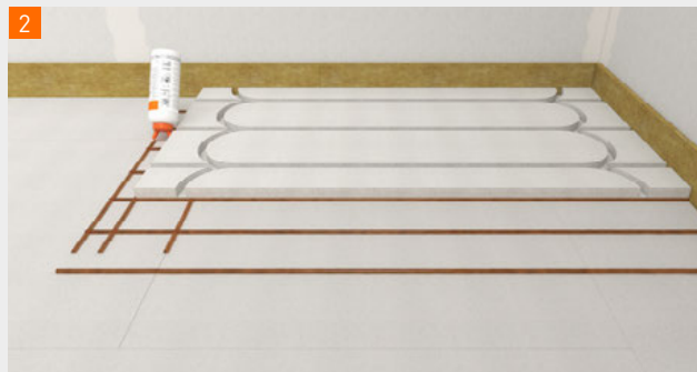
De lijmrillen voor de voegverlijming van het fermacell® Therm25™ element aanbrengen.
