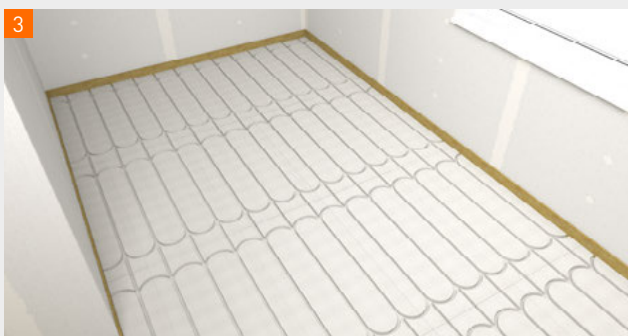
De ruimte dichtleggen met fermacell® Therm25™ elementen.
