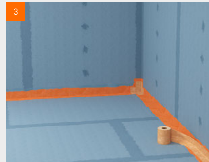
De fermacell™ afdichtband in de nog natte vloeibare folie drukken
