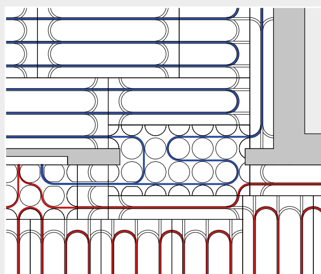
Voorbeeld van het plaatsingsschema bij een deuropening.
